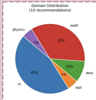
NeuMF
